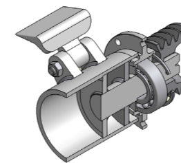
Μαχαιροφόρος άξονας St52 Ø168 Rotor shaft St52 Ø168
