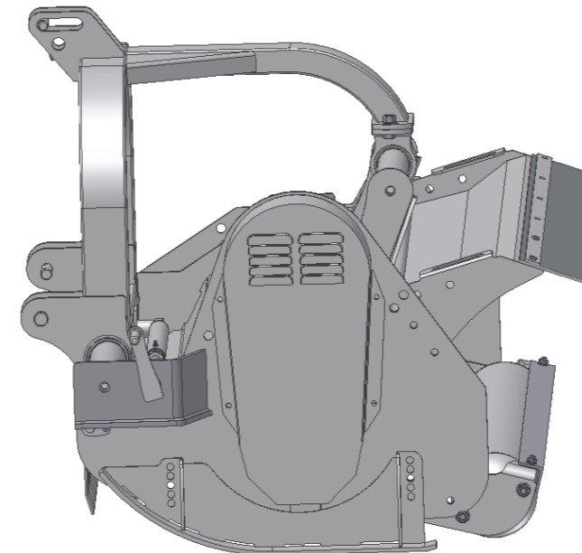
Με ρυθμιζόμενο ανοιγόμενο καπάκι With regulated back open cap
